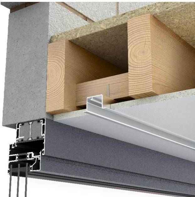
Inbouwprofiel
