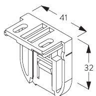
SG 10679 Steun kettingzijde
