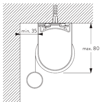
Bevestigingsprofiel SG 10534 en spanner SG 3033 of SG 3044
