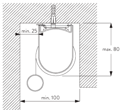
Bevestigingsprofiel SG 10534 en clicksteun SG 10539 Niet mogelijk met twee gekoppelde systemen!
