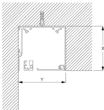
Bevestigingsprofiel SG 10534 en clicksteun SG 10539
