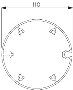
SG 4957 Profil ø 110 mm
