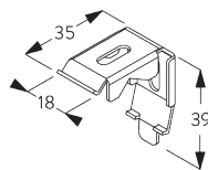
SG 2302 Plafondsteun
